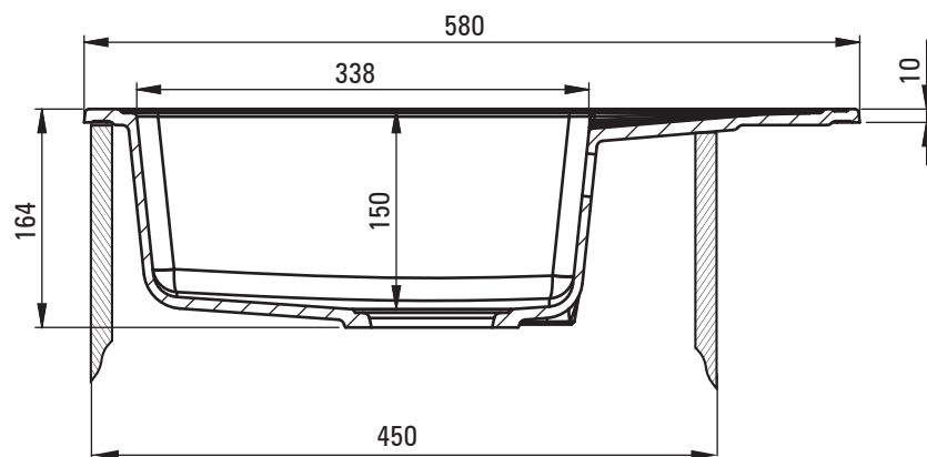
PRZEKRÓJ A-A
